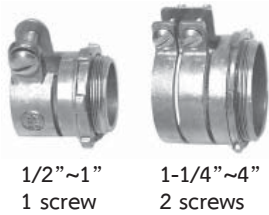
คอนเนคเตอร์จับท่ออ่อนเหล็ก Flexible Connectors
