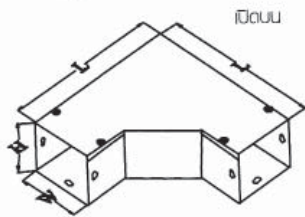
ข้องอ เปิดบน (HORIZONTAL ELBOW 90°)
