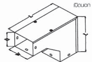
ข้องอ เปิดนอก (OUTSIDE VERTICAL)
